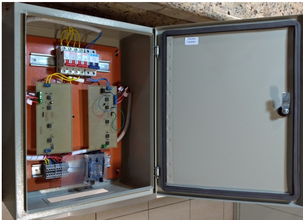
Figura 4.6: Painele com os dispositivos utilizados
