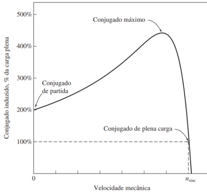
Figura 2.5: Curva característica de conjugado versus velocidade de um motor de indução típico. (CHAPMAN, 2013)
