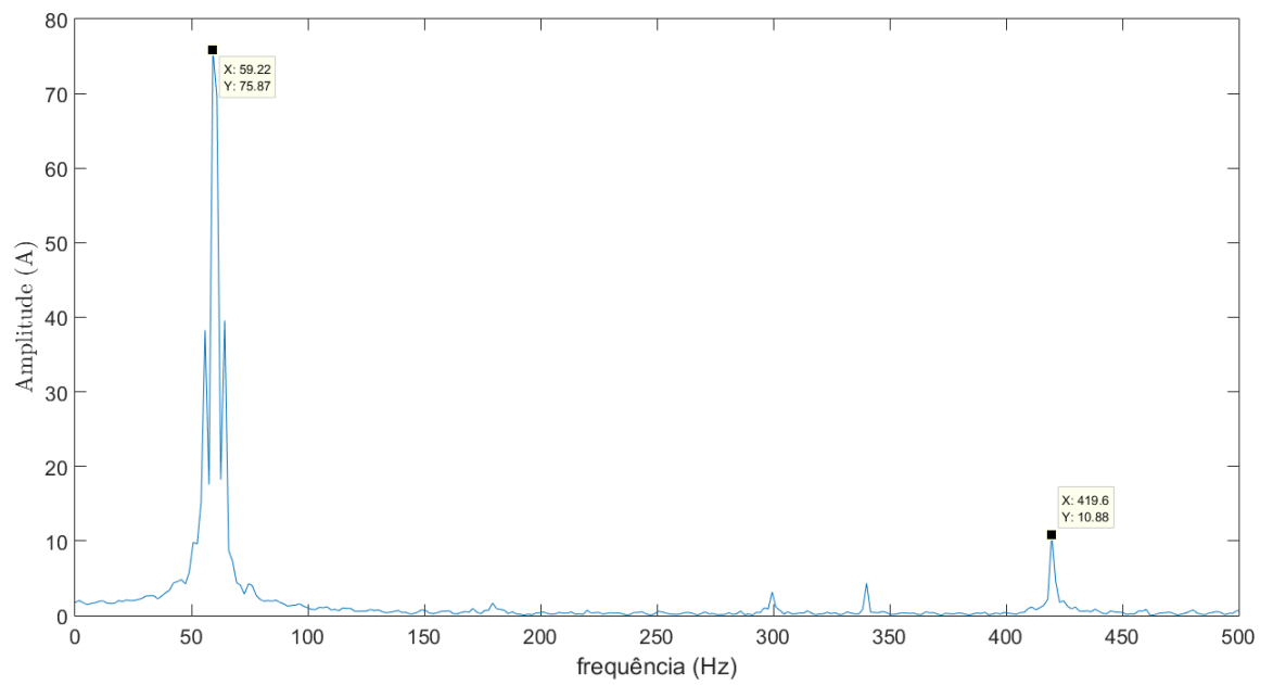
Figura 4.11: Amplitude do sinal de corrente após a implementação da FFT para o sinal de 0,6s
