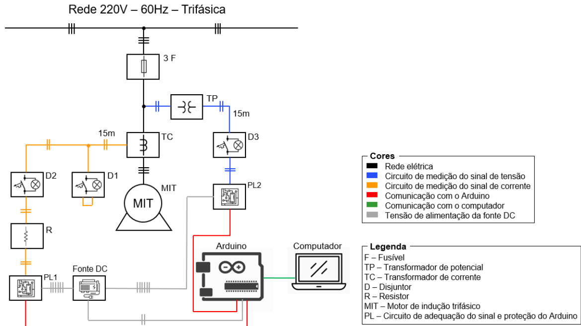
Figura 3.12: Diagrama unifilar do circuito medidor de potência ativa
