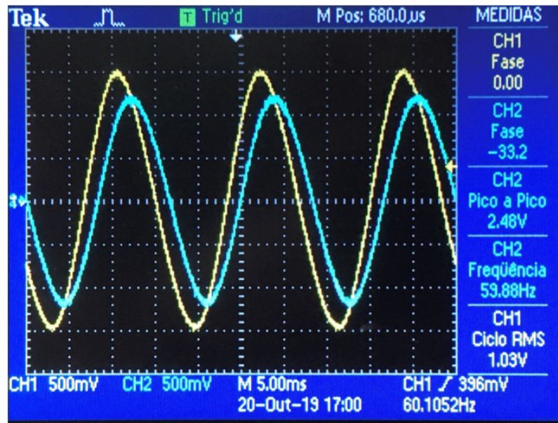
Figura 4.14: Sinal de validação do algoritmo visto através do osciloscópio
