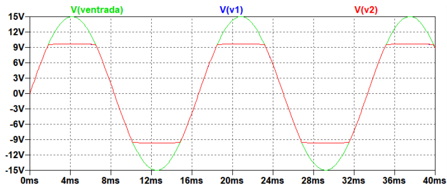
Figura 3.7: Comportamento do sinal após o buffer para V_{entrada} = 15V
