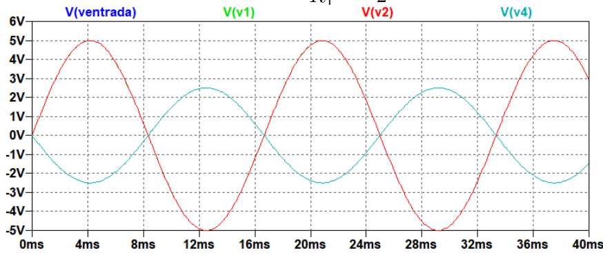
Figura 3.8: Sinal de saída V4 do amplificador operacional U2 para V_{entrada} = 5V
